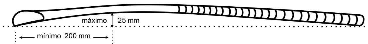
Figura 6: Dispositivo para medir el arco o inclinación del palo
